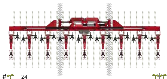
Voie 200 cm
