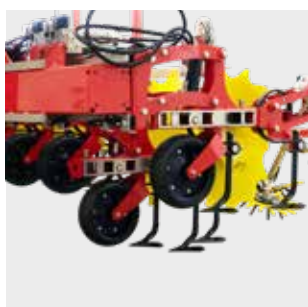
Relevage individuel électro-hydraulique
